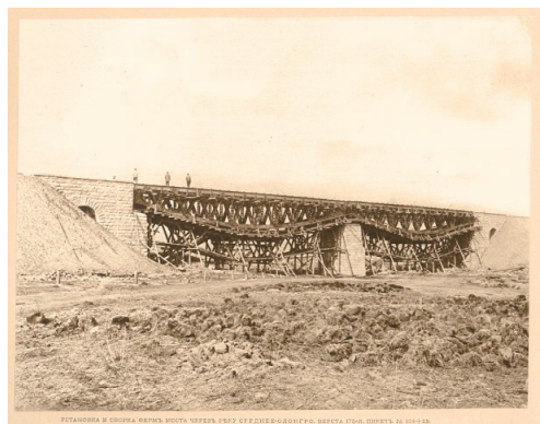
Установка и сборка ферм моста через р. Среднее Олонгро
