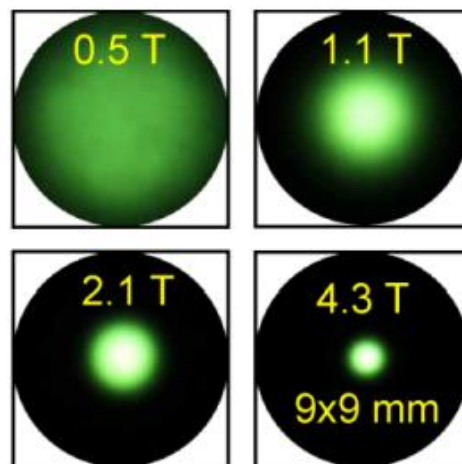
Рис.2. Структура пучка убегающих электронов на люминофоре
