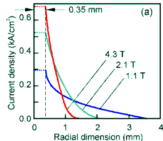
Рис.3. Распределение тока электронов по радиусу при различных магнитных полях
