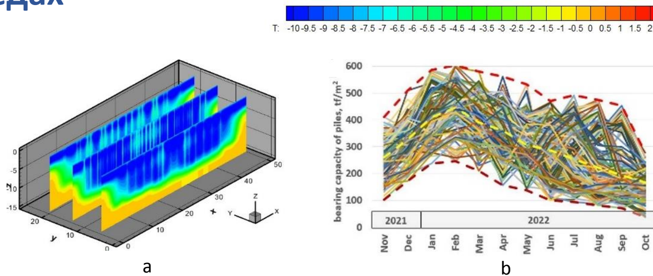
Температурные поля в области свайного фундамента жилого дома в Салехарде в марте 2021 г. (а); динамика изменения несущей способности свай (б) Тс/м 2
