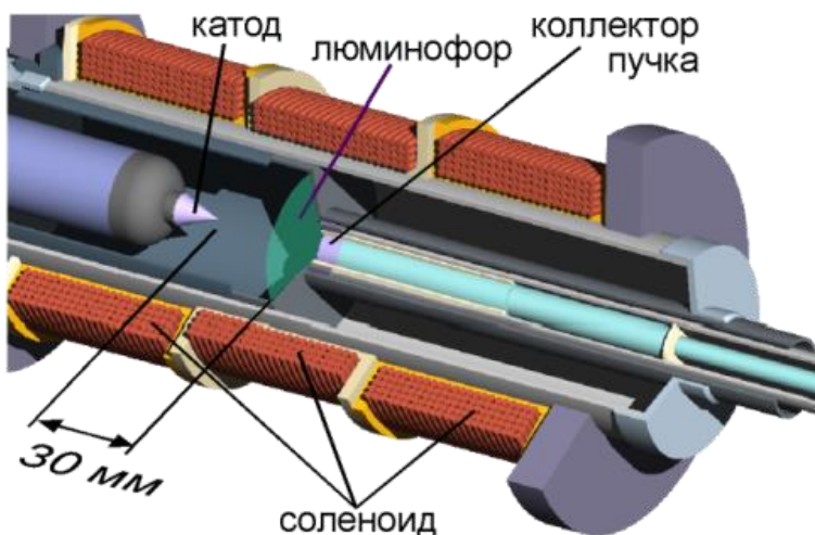
Рис.1. Геометрия атмосферного диода с конусным катодом и сильным продольным магнитным полем
